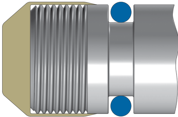
Montage d'un joint torique au-dessus d'un filetage
