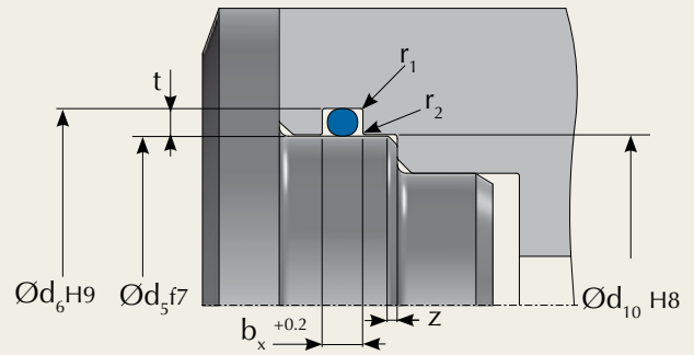
Montage radial Tige
