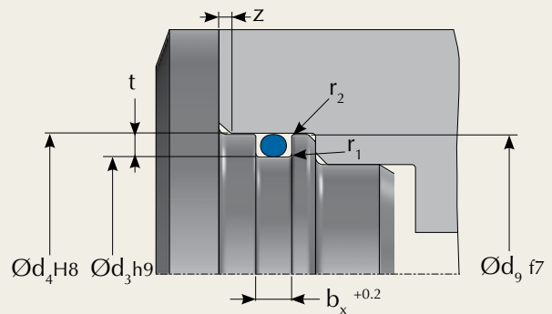
Montage radial Piston
