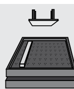
Positionnement des bandes sur la partie intermédiaire
