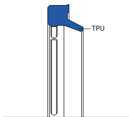
Composition d'un TDJR PU
