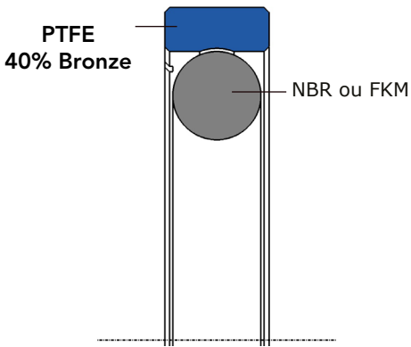
Composition d'un CPDE
