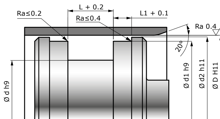
Préconisation de montage d'un JP3
