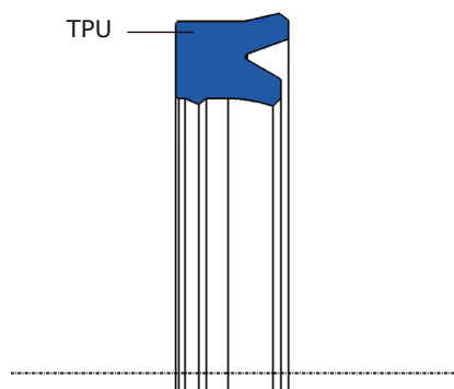
Composition d'un IDSL
