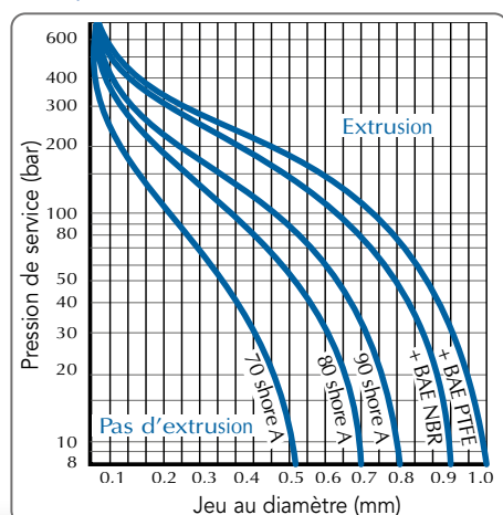
Abaque de sélection de dureté & de BAE
