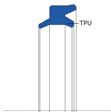
Composition d'un TDK DL PU
