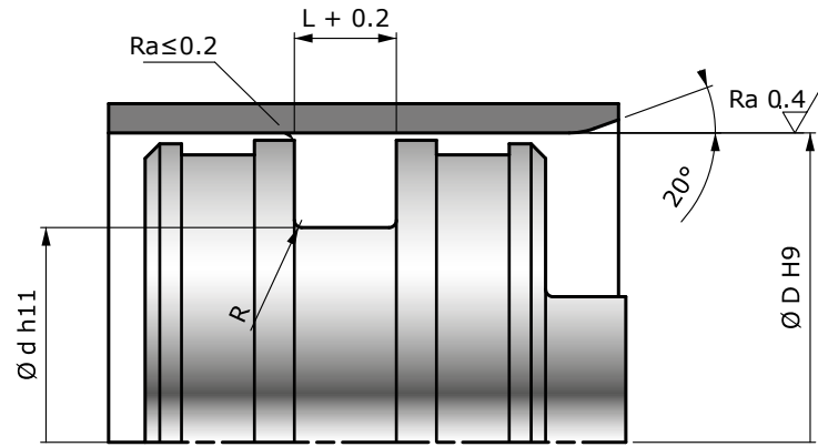
Préconisation de montage d'un CPDE
