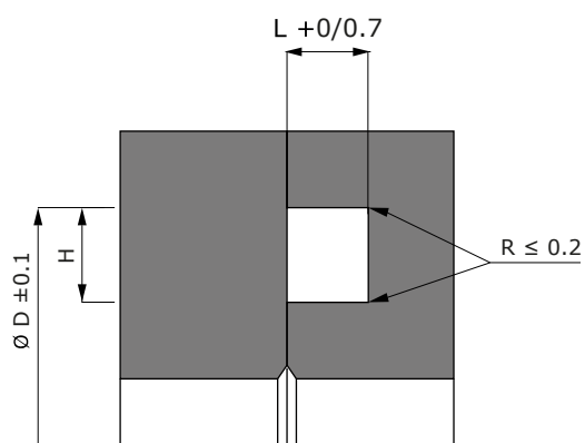
Préconisation de montage d'un BHS
