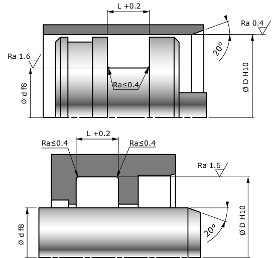
Préconisation de montage d'un UN
