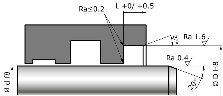
Préconisation de montage d'un TPA
