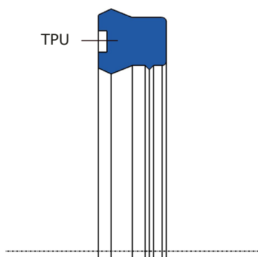
Composition d'un UM LR PU
