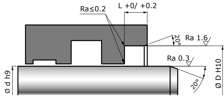
Préconisation de montage d'un TDJR NBR
