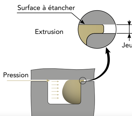
Principe de l'extrusion
