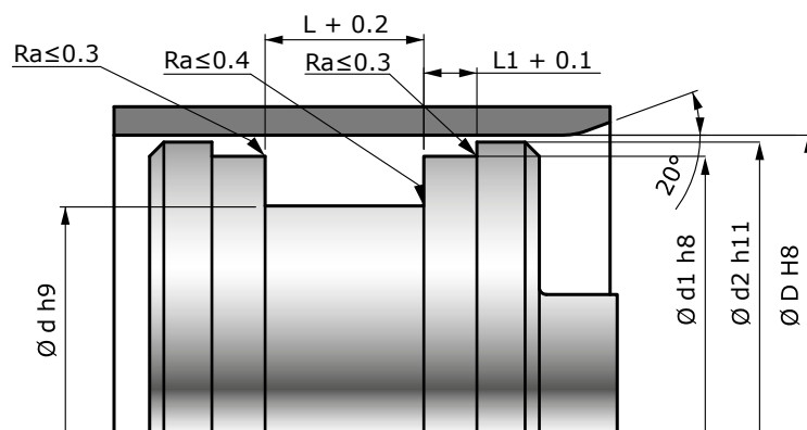
Préconisation de montage d'un JP5
