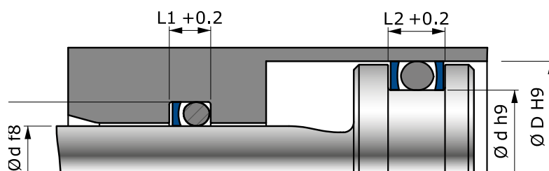
Préconisation de montage d'une bague anti-extrusion
