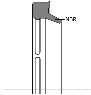
Composition d'un TDJR NBR
