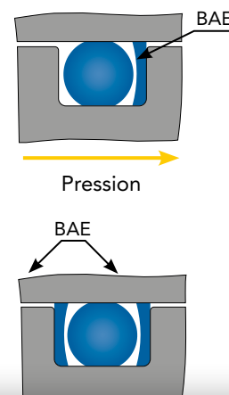
Positionnement des BAE suivant la pression
