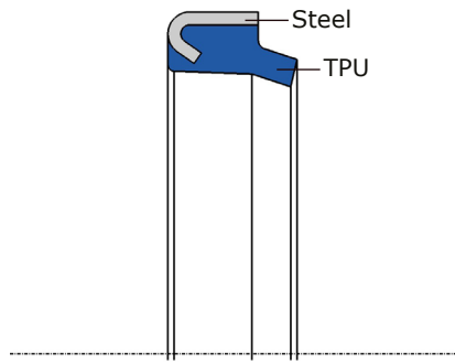
Composition d'un TPA
