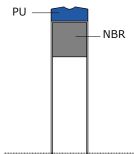
Composition d'un CPPU SR
