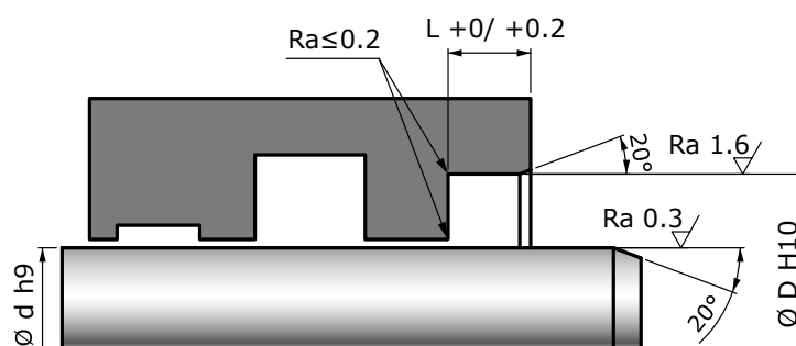
Préconisation de montage d'un TDJR PU
