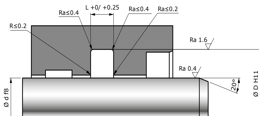
Préconisation de montage d'un UM LR PU
