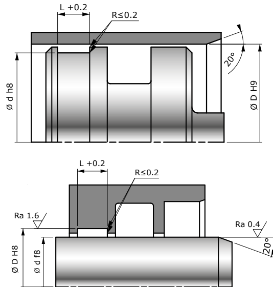
Préconisation de montage d'un segment de guidage
