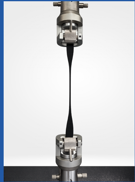
Essai de traction
