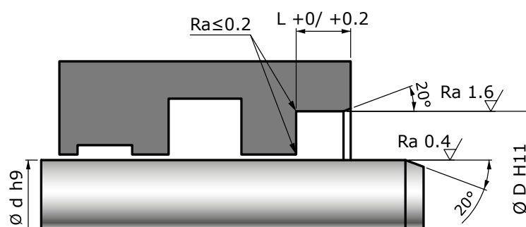
Préconisation de montage d'un TDK DL PU
