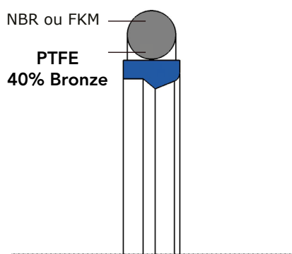
Composition d'un CTSE
