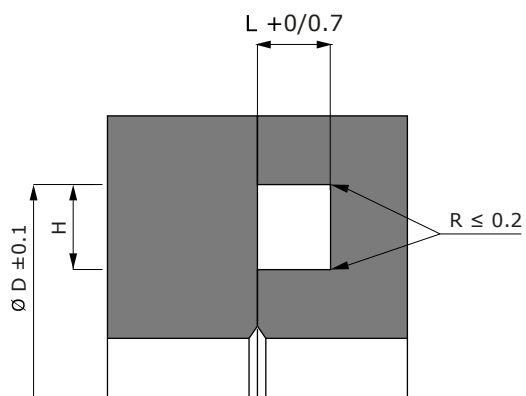
Préconisation de montage d'un SAE
