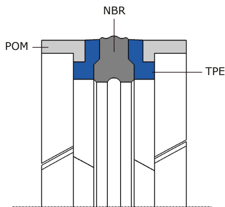
Composition d'un JP5
