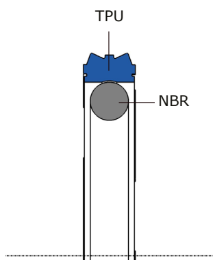
Composition d'un CPPU OR
