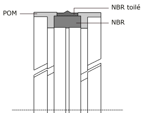
Composition d'un JP3
