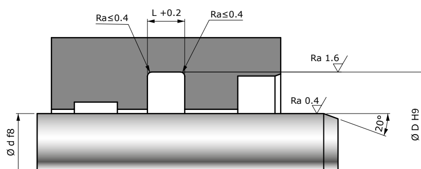
Préconisation de montage d'un CTSE
