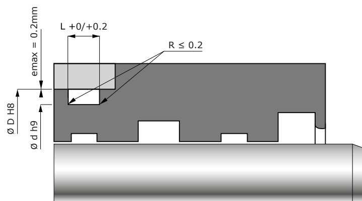
Préconisation de montage d'un OPPU
