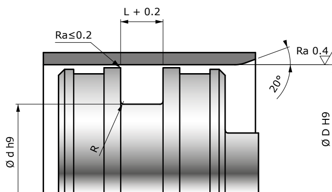
Préconisation de montage d'un CPPU SR
