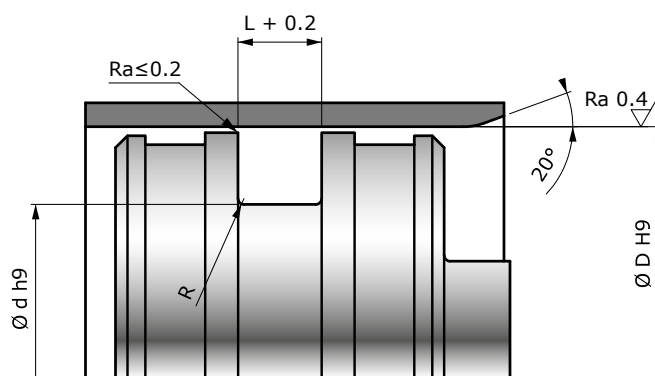
Préconisation de montage d'un CPPU OR
