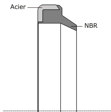
Composition d'un TRM
