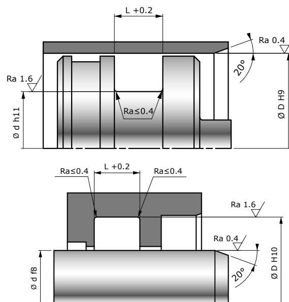
Préconisation de montage d'un TYPE B
