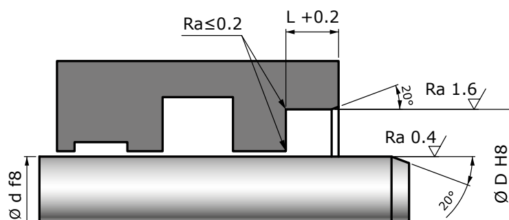
Préconisation de montage d'un TRM
