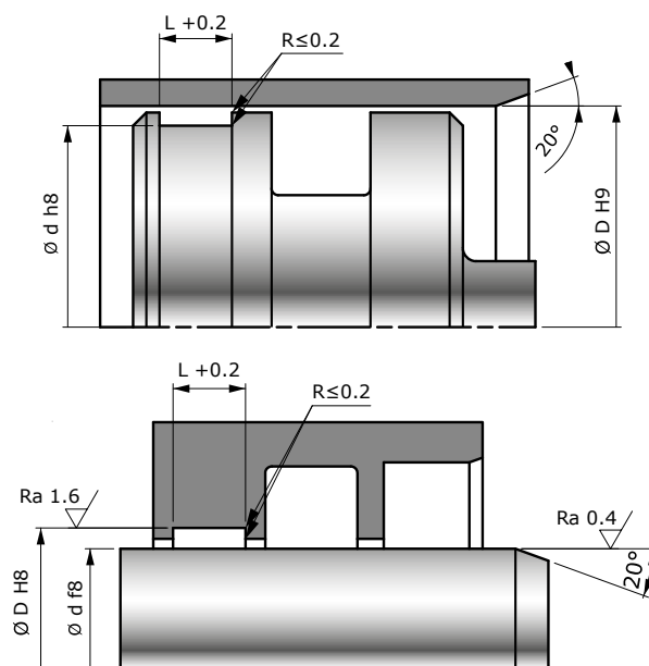
Préconisation de montage d'un TECBZ / TECKOT
