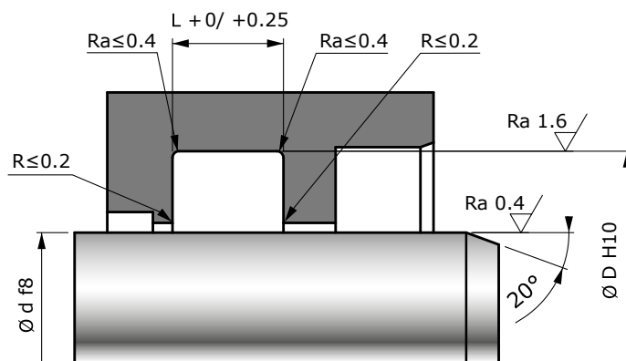
Préconisation de montage d'un IDSL
